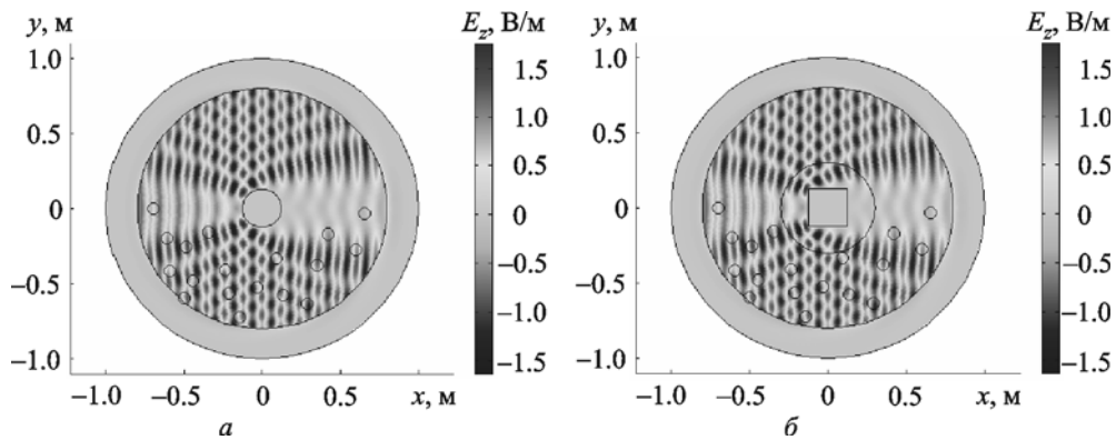
Рис. 6. Распределение z -компоненты электрического поля вблизи идеально проводящего кругового цилиндра (а) и вблизи плаща мимикрии цилиндра квадратного сечения под круговой (б)
