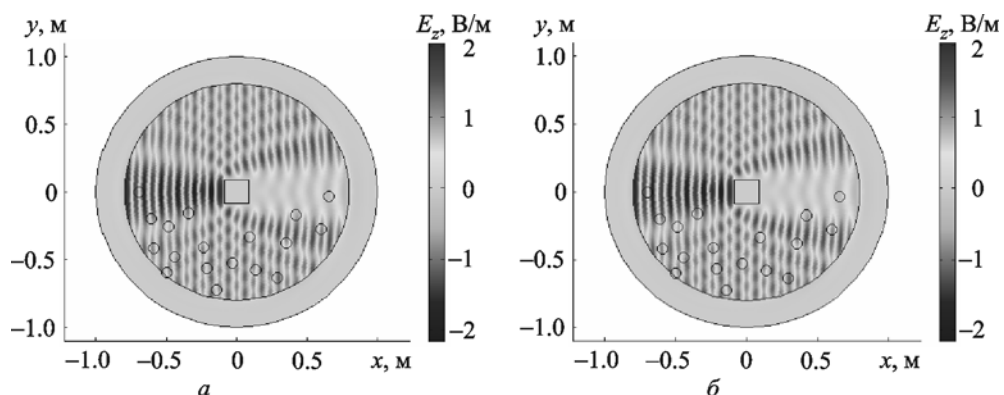
Рис. 7. Распределение z -компоненты электрического поля вблизи идеально проводящего цилиндра квадратного сечения (а) и вблизи плаща мимикрии кругового цилиндра под цилиндр квадратного сечения (б)
