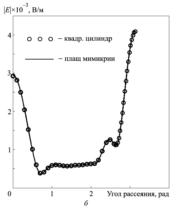
Рис. 5. Диаграммы рассеяния кругового цилиндра и плаща мимикрии цилиндра квадратного сечения под круговой (а) и цилиндра квадратного сечения и плаща мимикрии кругового цилиндра под цилиндр квадратного сечения (б)
