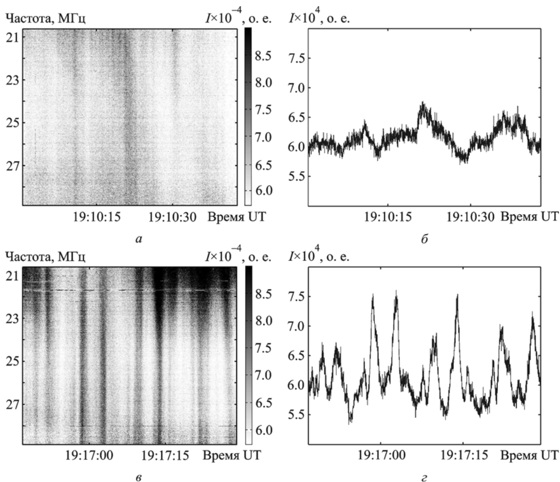
Рис. 2. Пример реализаций процесса мерцаний, которые были получены на радиотелескопе УТР-2 из наблюдений радиоисточника 3С144 вблизи 19:00 LT 17 и 18 февраля 2011 г.: a и c – динамические спектры мерцаний (интенсивность в зависимости от времени и частоты) 17 и 18 февраля соответственно, b и d – соответственно сечения этих динамических спектров на частоте 25 МГц
