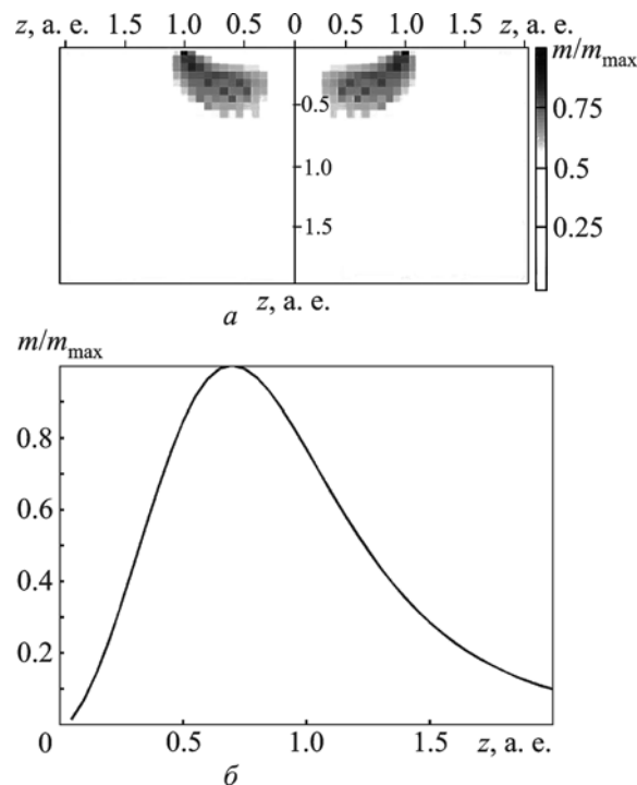
Рис. 5. Относительная эффективность слоев межпланетной плазмы: а – за орбитой Земли в плоскости эклиптики (0,0 – положение Земли, z – расстояние от Земли до рассеивающего слоя), б – в направлении на радиоисточник 3C144 ( \epsilon = 114^\circ )
