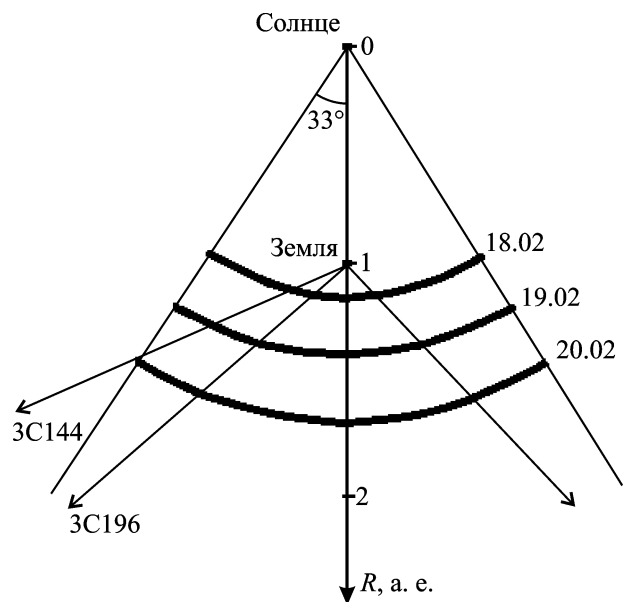
Рис. 6. Положение КВМ, произошедшего 15 февраля 2011 г., в межпланетном пространстве за орбитой Земли (жирные кривые) по наблюдениям межпланетных мерцаний 18, 19 и 20 февраля 2011 г.
