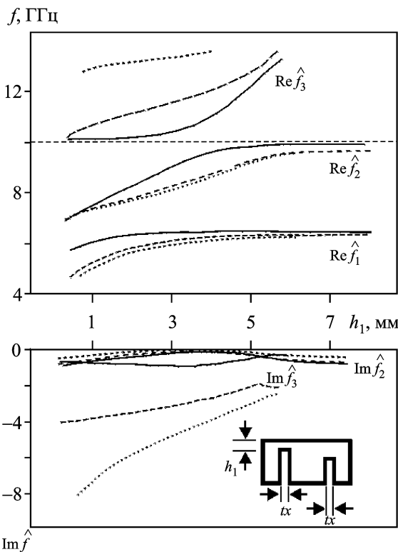
Рис. 4. Параметрические зависимости реальных и мнимых частей комплексных частот собственных колебаний Re \hat{f}'_1, Re \hat{f}'_2, Re \hat{f}'_3, Im \hat{f}'_1, Im \hat{f}'_2, Im \hat{f}'_3 = \varphi(h_1) при различных значениях ширины штырей: — — — tx = 0.5 мм, - - - - tx = 3.0 мм, ···· — tx = 4.0 мм
