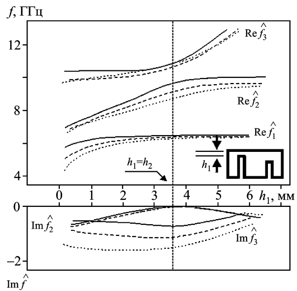
Рис. 5. Параметрические зависимости реальных и мнимых частей комплексных частот собственных колебаний Re \hat{f}'_1, Re \hat{f}'_2, Re \hat{f}'_3, Im \hat{f}'_1, Im \hat{f}'_2, Im \hat{f}'_3 = \varphi(h_1) при различных значениях ширины штырей: — — — t = 0.5 мм, - - - - t = 2.0 мм, ···· — t = 4.0 мм
