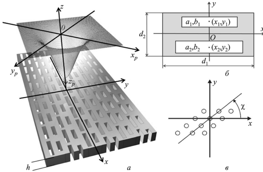
Рис. 1. Нормальное падение гауссова волнового пучка на двумерно-периодическую структуру (а), базовая ячейка структуры (б), косоугольная решетка (в)
