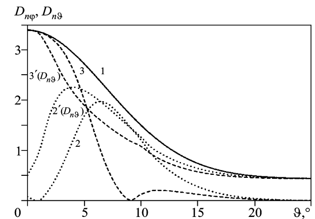
Рис. 6. Диаграммы направленности по полю падающего (кривая 1), прошедшего (кривые 2 и 2' (D_{n\theta}) ) и отраженного (кривые 3 и 3' (D_{n\theta}) ) пучков при \lambda = 7.055 мм
