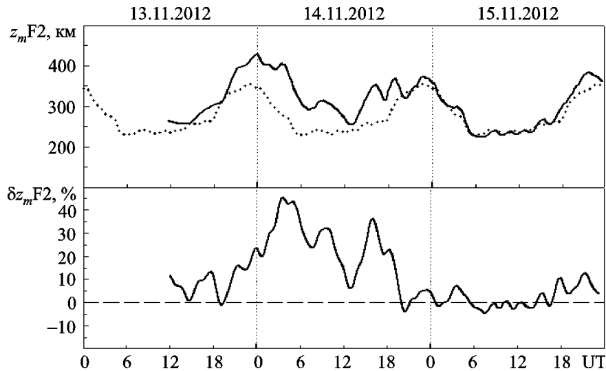
Рис. 3. Временные вариации высоты максимума слоя F2, z_mF2 , (верхняя панель, сплошная линия), а также ее относительно отклонения \delta z_mF2 , % (нижняя панель) с 13 по 15 ноября 2012 г. Пунктирная линия на верхней панели – данные в контрольный день 22 ноября 2012 г.
