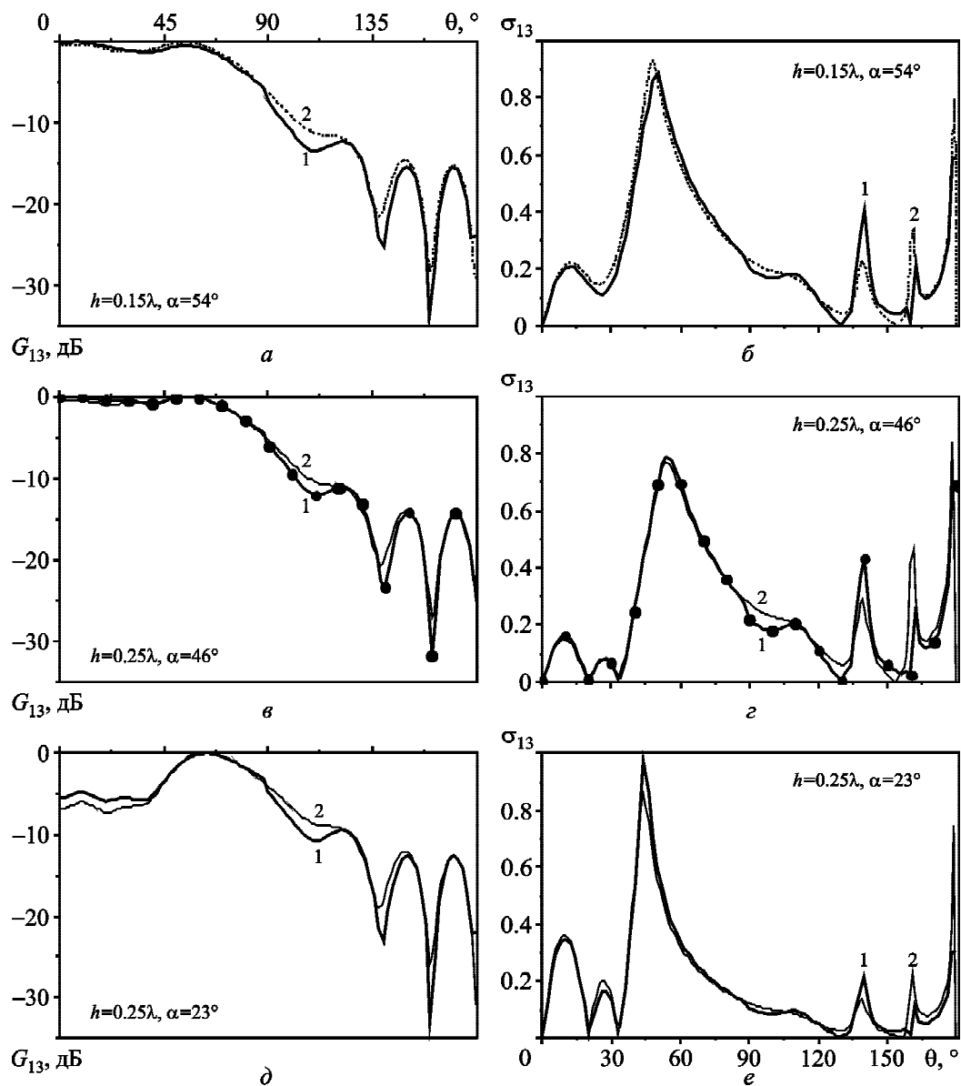
Рис. 7. К сравнению ДН по мощности ( a , в , д ) и поляризационных ДН ( б , з , е ) наклонного полуволнового вибратора, расположенного над квадратным экраном с размерами W = L = 3\lambda , рассчитанных методом РГТД (кривые 1) и методом моментов (кривые 2) в плоскости наблюдения \varphi = 90^\circ
