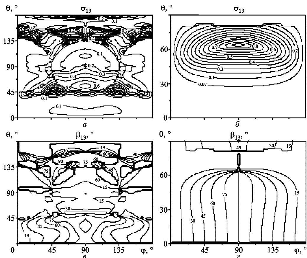
Рис. 8. Линии равных значений коэффициентов эллиптичности \sigma_{13} и углов ориентации \beta_{13} векторов полного (а, в) и ГО (б, з) полей в системе координат (\theta, \varphi) в случае, когда вибратор с углом наклона \alpha = 46^\circ и током I_{13} находится над серединой экрана с размерами W = L = 3\lambda при h = 0.25\lambda .
