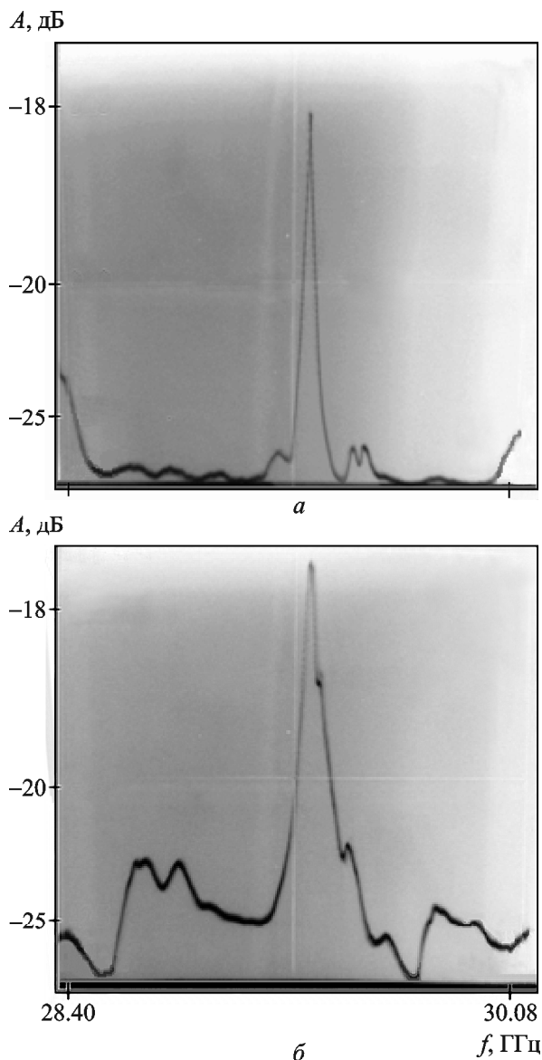
Рис. 2. Участки спектров колебаний двухслойных экранированных ДР на основе диэлектрических диска (а) и полушара (б)
