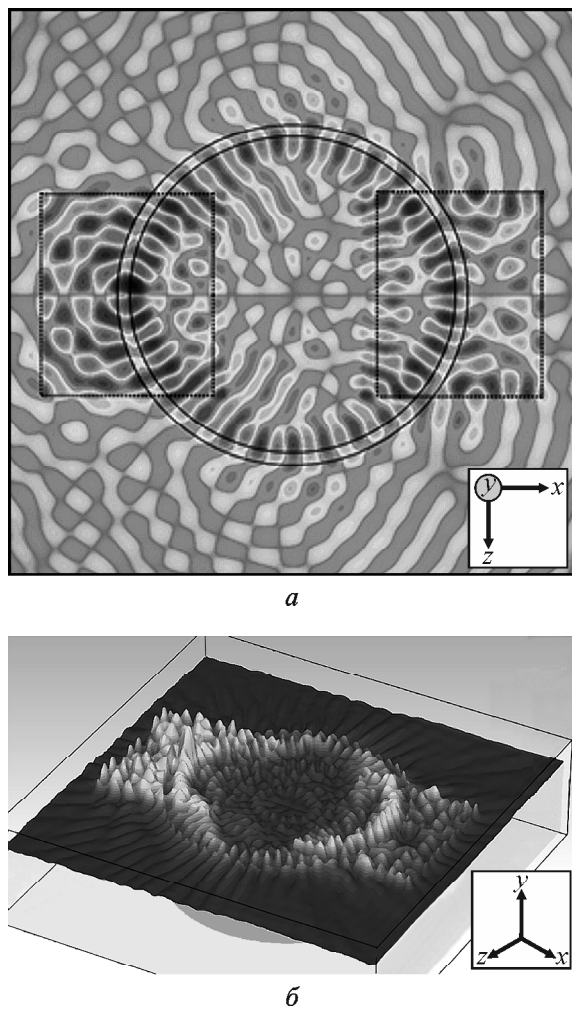
Рис. 3. Распределение поля HE_{3111} -моды ШГ в экранированном дисковом ДР
