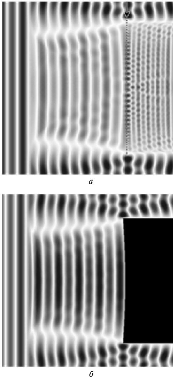
Рис 5. Пространственное распределение электрического поля при падении плоских волн на градиентную металлическую решетку (а) и вогнутое металлическое зеркало (б)
