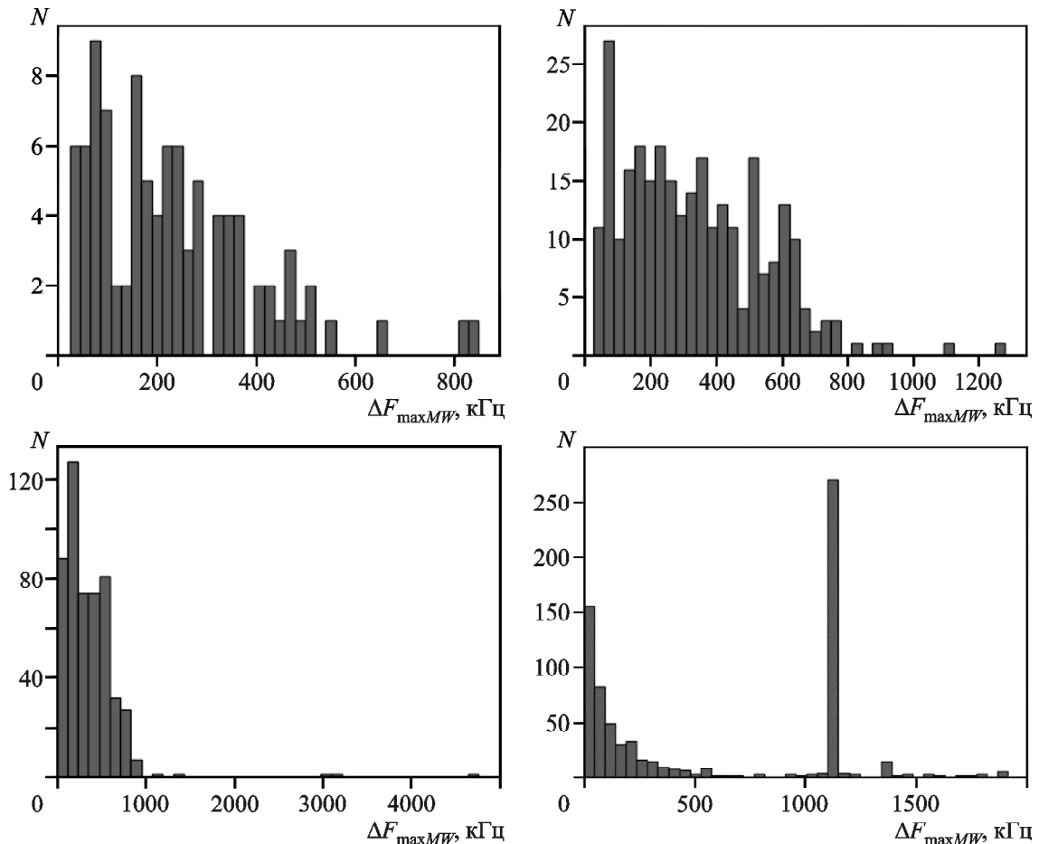
Рис. 6. Гистограммы распределения мазерных линий: линии ОН вблизи частоты 6 ГГц (верхняя левая панель), линии \text{CH}_3\text{OH} вблизи частоты 6.7 ГГц (верхняя правая панель, нижняя левая панель), линии \text{H}_2\text{O} вблизи частоты 22 ГГц (нижняя правая панель), – в рабочей полосе частот радиотелескопа
