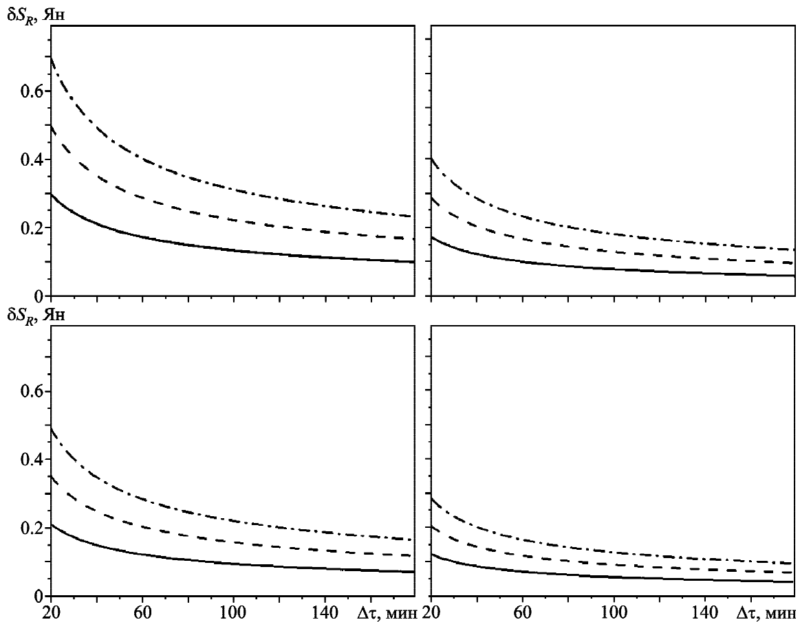
Рис. 5. Зависимость флуктуационной чувствительности радиотелескопа \delta S_R(f, \varphi_{El}) , которая достигается при измерении спектральной плотности потока, от времени накопления \Delta\tau в частотной полосе \Delta f = 1 \text{ кГц} (справа) и \Delta f = 3 \text{ кГц} (слева) для трех значений шумовой температуры системы: сплошная линия – T_{SN} = 30 \text{ К} , штриховая линия – T_{SN} = 50 \text{ К} , штрихпунктирная линия – T_{SN} = 70 \text{ К} . Верхние панели – \alpha = \sqrt{2} , нижние панели – \alpha = 1
