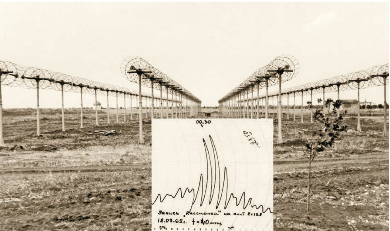
Рис. 2. Перший в Україні 24-елементний радіотелескоп декаметрових хвиль ID-1(2) діапазону 10 ÷ 25 МГц, споруджений в обсерваторії поблизу с. Гракове Харківської обл. на початку 60-х років
