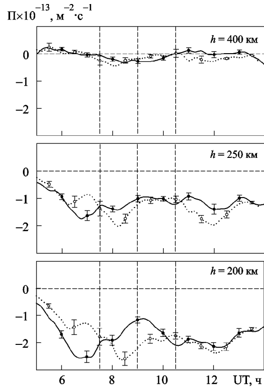
Рис. 6. Временные вариации плотности потока плазмы \Pi на фиксированных высотах в день затмения 4 января (сплошные линии) и в контрольный день 5 января 2011 г. (точки)
