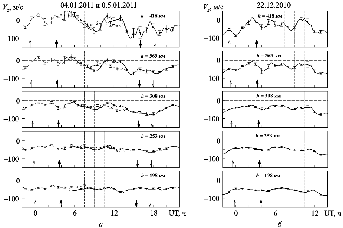
Рис. 2. Временные вариации вертикальной составляющей скорости движения ионосферной плазмы V_z на фиксированных высотах (скользящее усреднение на интервале 75 мин с шагом 15 мин): а – в день затмения 4 января (сплошные линии) и контрольный день 5 января (точки) 2011 г.; б – в контрольный день 22 декабря 2010 г. Жирными стрелками обозначены моменты восхода и захода Солнца на соответствующих высотах в Харькове, а тонкими – в магнитосопряженной точке. Вертикальные пунктирные линии здесь и на последующих рисунках обозначают моменты, соответствующие началу, главной фазе и окончанию СЗ
