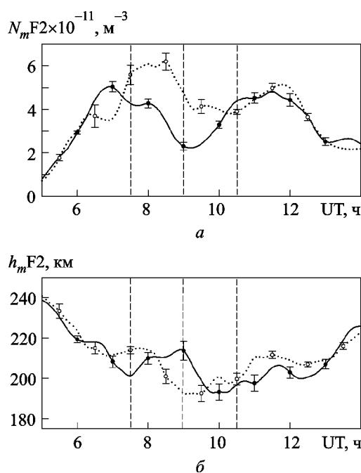
Рис. 5. Временные вариации концентрации электронов N_m F2 в максимуме слоя F2 ионосферы (а) и высоты h_m F2 максимума ионизации (б) в день затмения 4 января (сплошные линии) и в контрольный день 5 января 2011 г. (точки)
