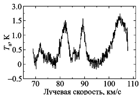
Рис. 4. Спектр излучения молекулы ^{13}CO на переходе J = 1 - 0 (110.201 ГГц) в направлении источника G33.6+0.1, полученный в режиме диаграммной модуляции фурье-анализатором спектра. Время накопления полезного сигнала 250 с
