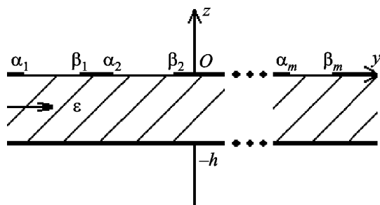
Рис. 1. Геометрия структуры и система координат
