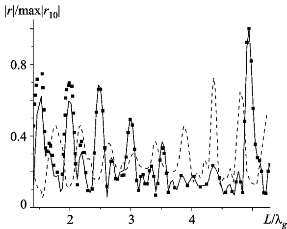
Рис. 3. Зависимость нормированного коэффициента отражения волны H_{01} (сплошная линия) и H_{02} (пунктирная линия) от параметра L/\lambda_g для структуры из четырех эквидистантно расположенных щелей при k_1h = 6 , k_1d = 6 , \epsilon = 2.4 . Маркерами обозначены результаты, полученные операторным методом для волны H_{01}
