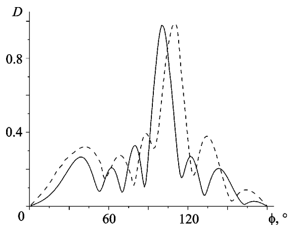
Рис. 5. Нормированные диаграммы направленности D(\phi) для структур из четырех щелей
