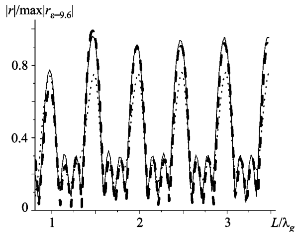
Рис. 2. Зависимость нормированного коэффициента отражения от параметра L/\lambda_g для структуры из четырех эквидистантно расположенных щелей при k_1 h = 6 , k_1 d = 6 : \epsilon = 1 – линия из точек; \epsilon = 2.4 – сплошная линия; \epsilon = 9.6 – пунктирная линия
