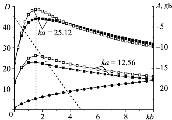
Рис. 3. Залежність КС лінзової антени (ліва вісь) та параметра освітлення краю (права вісь) від ширини хвильового пучка, що випромінюється КД: —●— — D_e ; —□— — E -поляризація; —■— — H -поляризація. Параметри лінзи: l_1 = 0.8 , l_2 = 1.286 , \epsilon = 2.53
