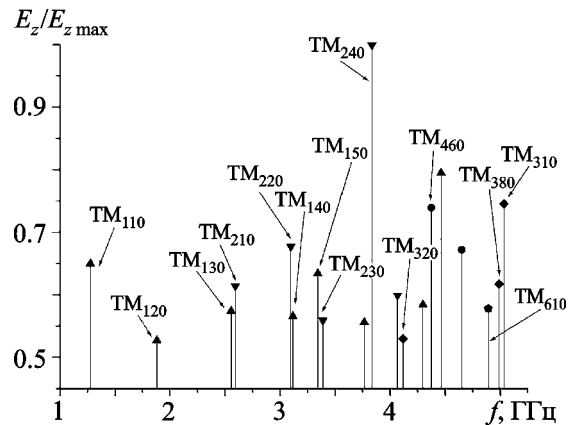
Рис. 3. Гистограмма спектра возбуждаемых колебаний при W_{\text{эфф}}/r_m = 0.5
