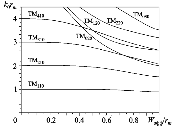
Рис. 2. Зависимость нормированных резонансных частот от параметра W_{\text{эфф}}/r_m
