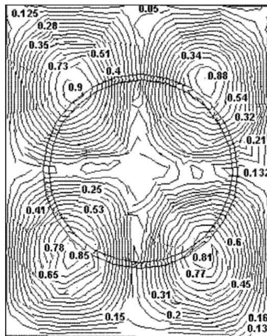
Рис. 5. Структура изолиний поля TM_{240} вида колебаний
