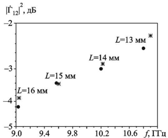
Рис. 6. Расчетные и экспериментальные резонансные значения коэффициента прохождения: ● – эксперимент, * – расчет
