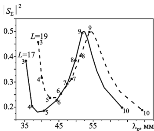
Рис. 5. Резонансные значения коэффициента излучения и резонансные длины волн при различных t , \epsilon = 7
