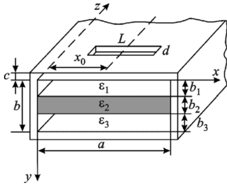
Рис. 1. Геометрия системы
