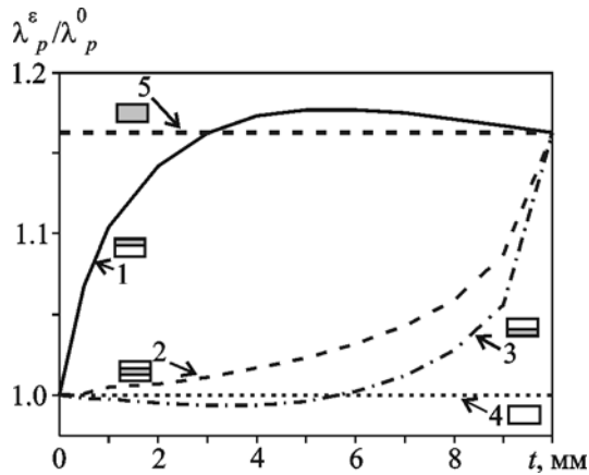
Рис. 2. Зависимость \lambda_p^\epsilon / \lambda_p^0 от толщины t диэлектрической пластины, \epsilon = 2 , для различных вариантов ее расположения в волноводе
