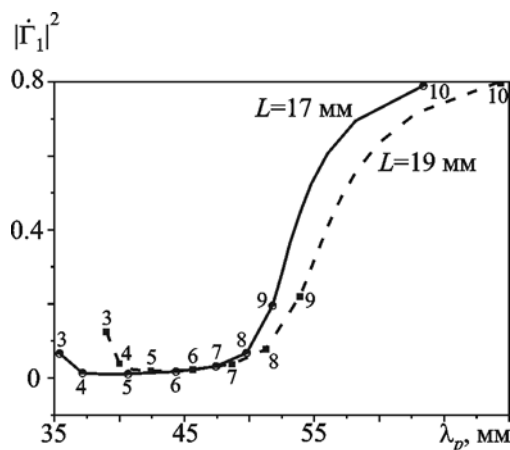
Рис. 4. Резонансные значения коэффициента отражения и резонансные длины волн при различных t , \epsilon = 7
