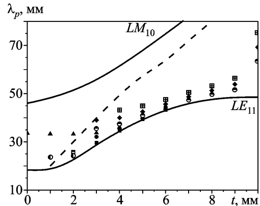
Рис. 3. Границы рабочей полосы и резонансные длины волн щелей разной длины в зависимости от толщины слоя t с \epsilon = 7 : \circ – L = 11 мм, \square – L = 12 мм, \blacksquare – L = 13 мм, \bullet – L = 15 мм, \blacktriangle – L = 16 мм, \odot – L = 17 мм, \blacklozenge – L = 19 мм, \boxplus – L = 21 мм
