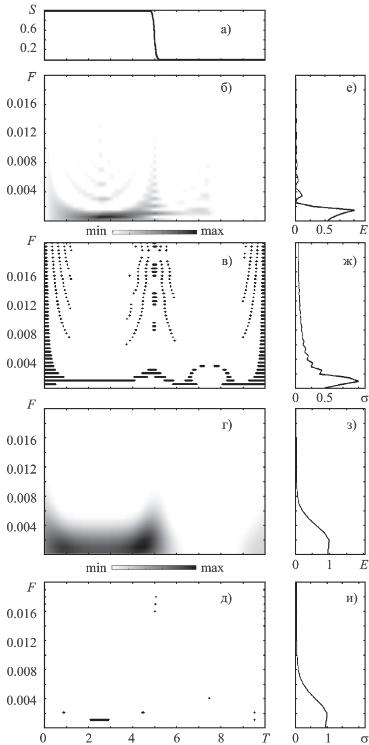
Рис. 1. Результаты анализа УВ, описываемой уравнением Бюргера: а) – УВ во временной области, б) – ФСП ПВ, в) – хребты ФСП ПВ, г) – ФСП СФ, д) – хребты ФСП СФ, е) – энергограмма ПВ, ж) – среднеквадратичное отклонение ФСП ПВ, з) – энергограмма СФ, и) – среднеквадратичное отклонение ФСП СФ
