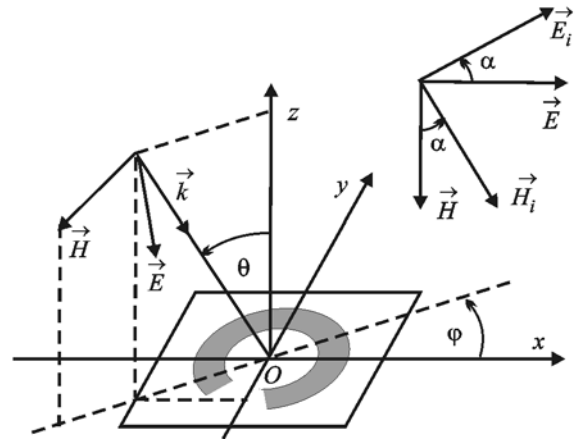
Рис. 2. Пространственная ориентация векторов электромагнитного поля в падающей волне. Показан случай падения TE-волны
