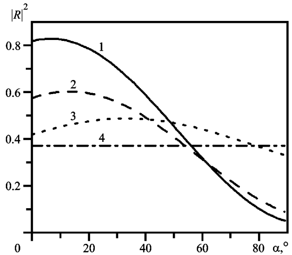
Рис. 7. Зависимости квадратов модулей коэффициентов отражения от угла поляризации падающей волны: линия 1 – \beta = 30^\circ ; линия 2 – \beta = 60^\circ ; линия 3 – \beta = 80^\circ ; линия 4 – \beta = 90^\circ
