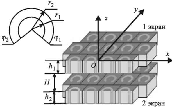
Рис. 1. Двойной экран конечной толщины с коаксиально-секторными отверстиями
