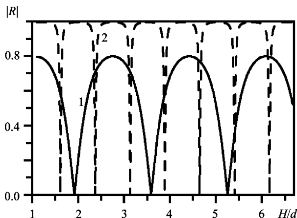
Рис. 4. Зависимости модуля коэффициента отражения от относительного расстояния между экранами: кривая 1 – d/\lambda = 0.3 ; кривая 2 – d/\lambda = 0.66
