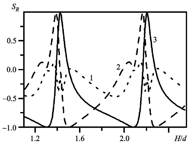
Рис. 8. Зависимости параметров Стокса отраженной волны от относительного расстояния между экранами: кривая 1 – S_1 ; кривая 2 – S_2 ; кривая 3 – S_3
