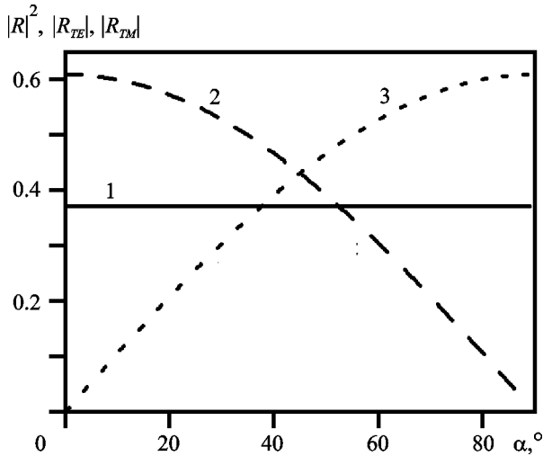
Рис. 6. Зависимости квадрата модуля коэффициента отражения (линия 1) и модулей коэффициентов отражения TE - и TM -волн (линия 2 и линия 3 соответственно) от угла поляризации падающей волны
