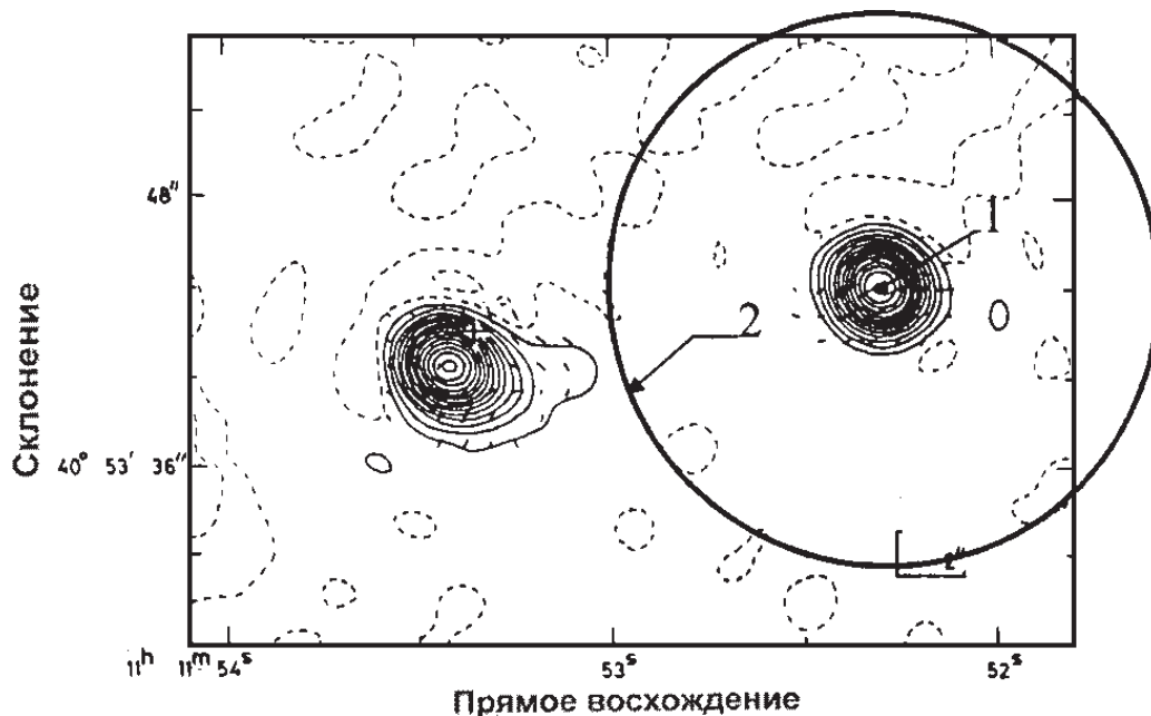
Рис. 4. Оптимальная простейшая модель распределения радиояркости 3C254 типа “ядро-галло” для декаметрового диапазона волн на фоне радиокарты источника на частоте 5 ГГц: 1 – компактный юго-западный компонент, 2 – протяженный компонент (галло)
