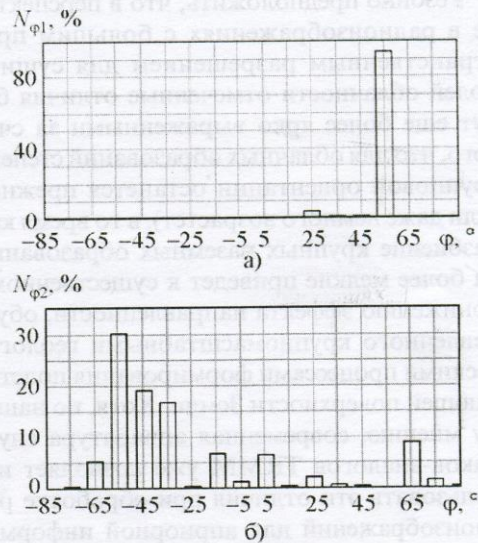
Рис. 5. Процентное распределение азимутальных углов ориентации контрастирующих сегментов на спутниковых радиотепловых изображениях (85 ГГц):
