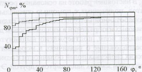
Рис. 6. Процентное распределение средних углов ориентации контрастирующих сегментов N_{\varphi} для обобщенных спутниковых радиотепловых изображений: верхняя кривая – усреднение для полей облачности над пятью регионами Атлантического, Тихого и Индийского океанов; нижняя кривая – усреднение для поверхности суши пяти регионов в Южной Америке, Южной Африке и Австралии
