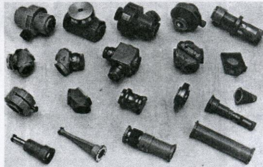
Комплект квазиоптических измерительных устройств на основе полого диэлектрического лучевода. Разработка ИРЭ. Фотография любезно предоставлена В. К. Киселевым (ИРЭ)
