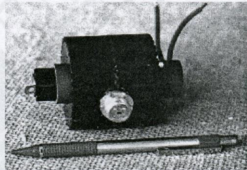
Магнетрон на пространственной гармонике с холодным катодом, импульсная мощность – 1 кВт, рабочая частота – 95 ГГц. Разработка РИ. Фотография любезно предоставлена Д. М. Вавривым (РИ)
