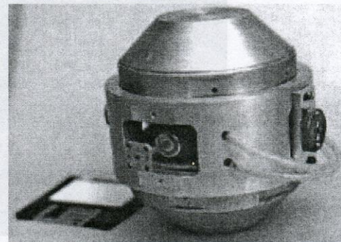
Клиноотрон, диапазон рабочих частот – 440 + 510 ГГц, выходная мощность – 50 мВт. Фотография любезно предоставлена Д. М. Вавривым (РИ)
