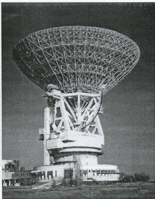
Антенная система RT-70 Национального центра управления и испытаний космических средств НКАУ. Фотография любезно предоставлена А. А. Коноваленко (РИ)
