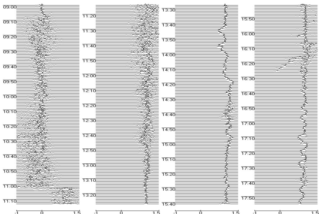
Рис. 3. Вариации доплеровских спектров в день ЗС, 11 августа 1999 г. ( f \approx 3.5 МГц). День относился к невозмущенным. Оси те же, что на рис. 1. В 11:13 введено смещение +1 Гц
